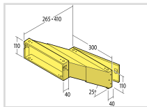
Briefkasten- anlage Nr. 9
